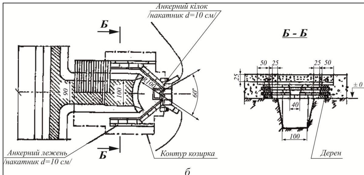
Рис. 5. Окоп з протиосколковим покриттям для стрільби з кулемета:
