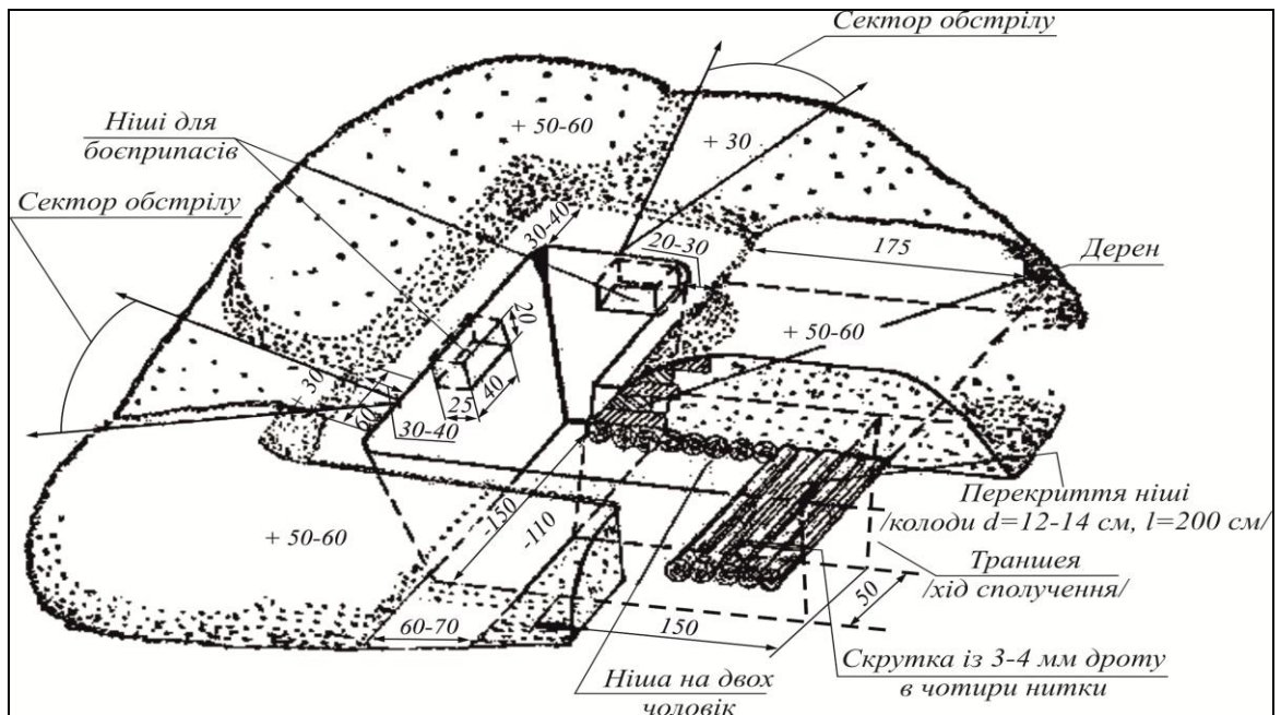
Рис. 3. Окоп для двох стрільців
