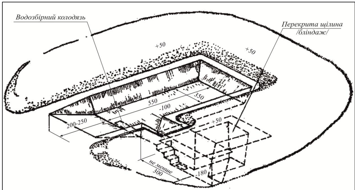
Рис. 9. Окоп для бойової машини піхоти з круговим обстрілом
