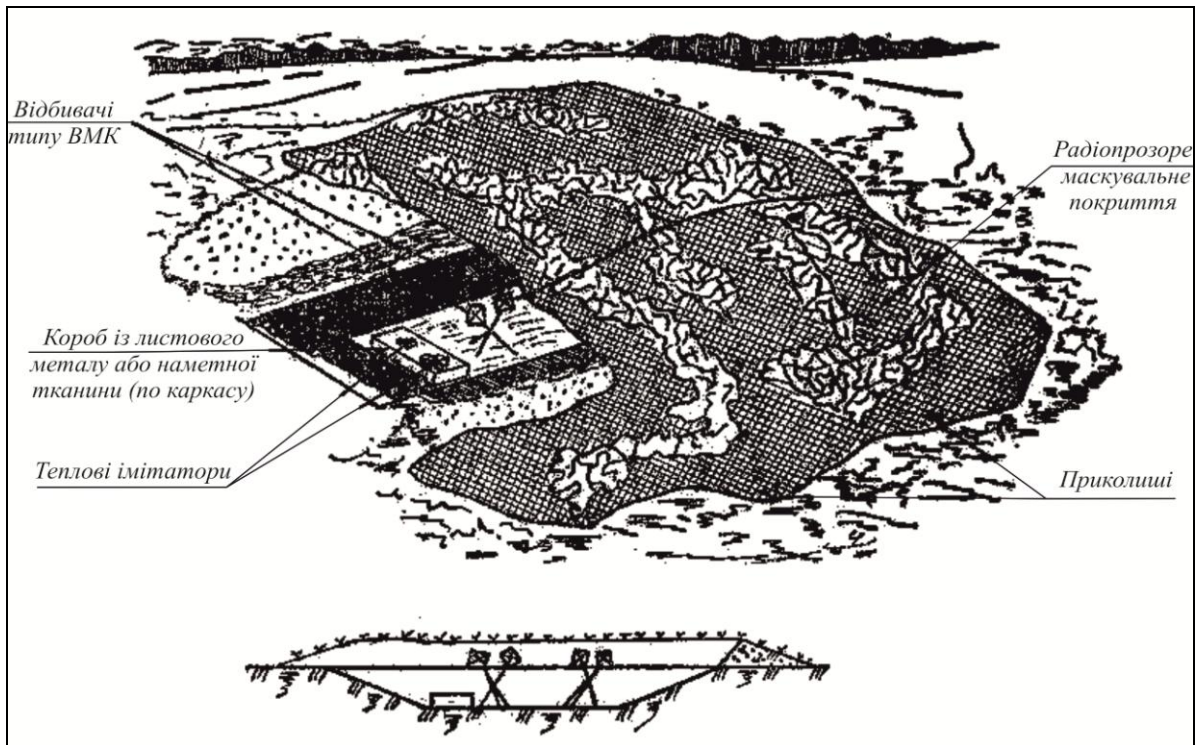
Рис. 21. Імітація техніки в укритті (окопі) із застосуванням маскувальних засобів
