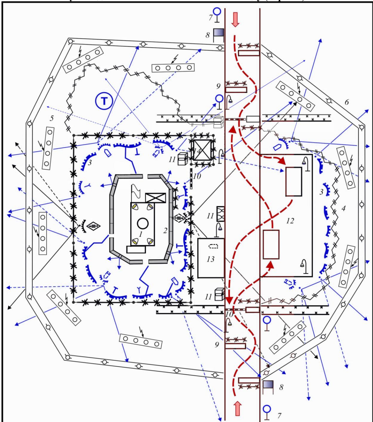
Схема блокпоста у складі посиленого механізованого взводу (варіант)
