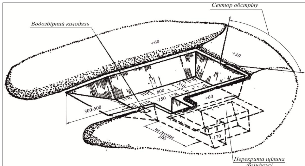
Рис. 11. Окоп для бронетранспортера
