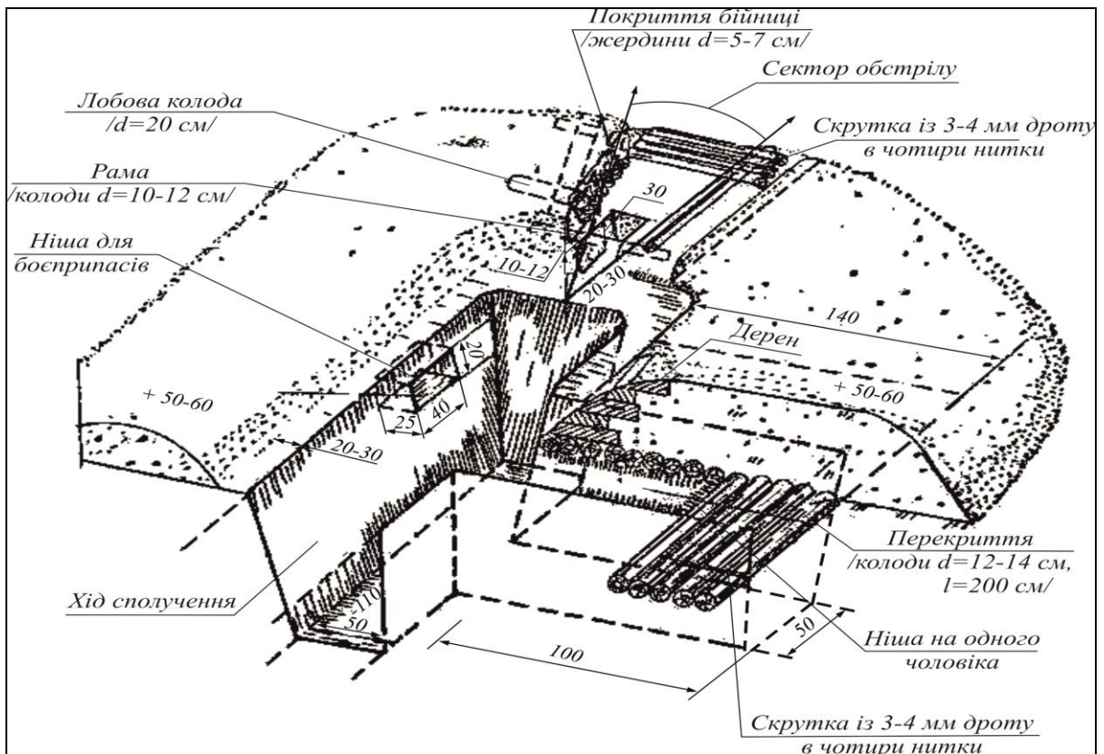
Рис. 4. Винесений окопчик для стрільця з нішею та перекритою бійницею
