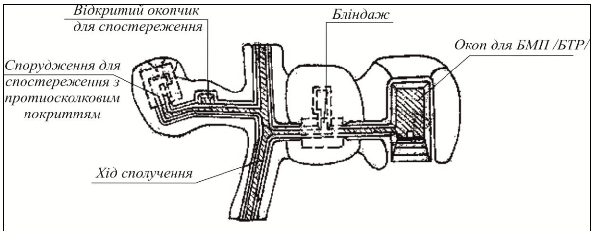
Рис. 17. Фортифікаційне обладнання КСП взводу
