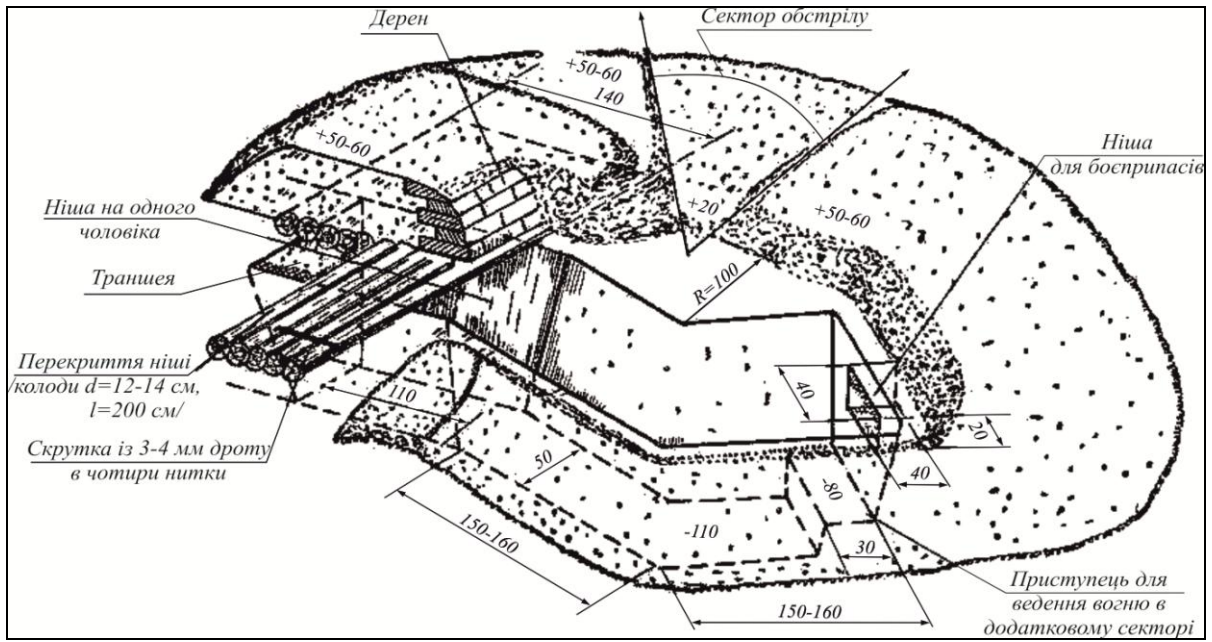
Рис. 6. Окоп для стрільби із кулемета стоячи
