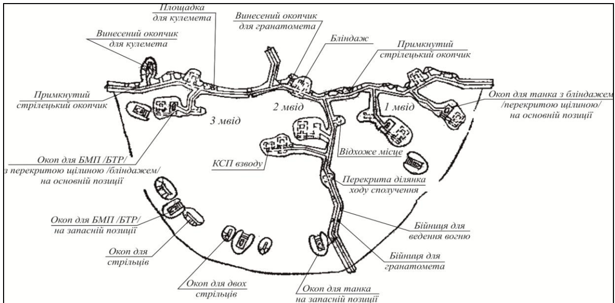
Рис. 19. Фортифікаційне обладнання опорного пункту механізованого взводу другого ешелону роти (варіант)
