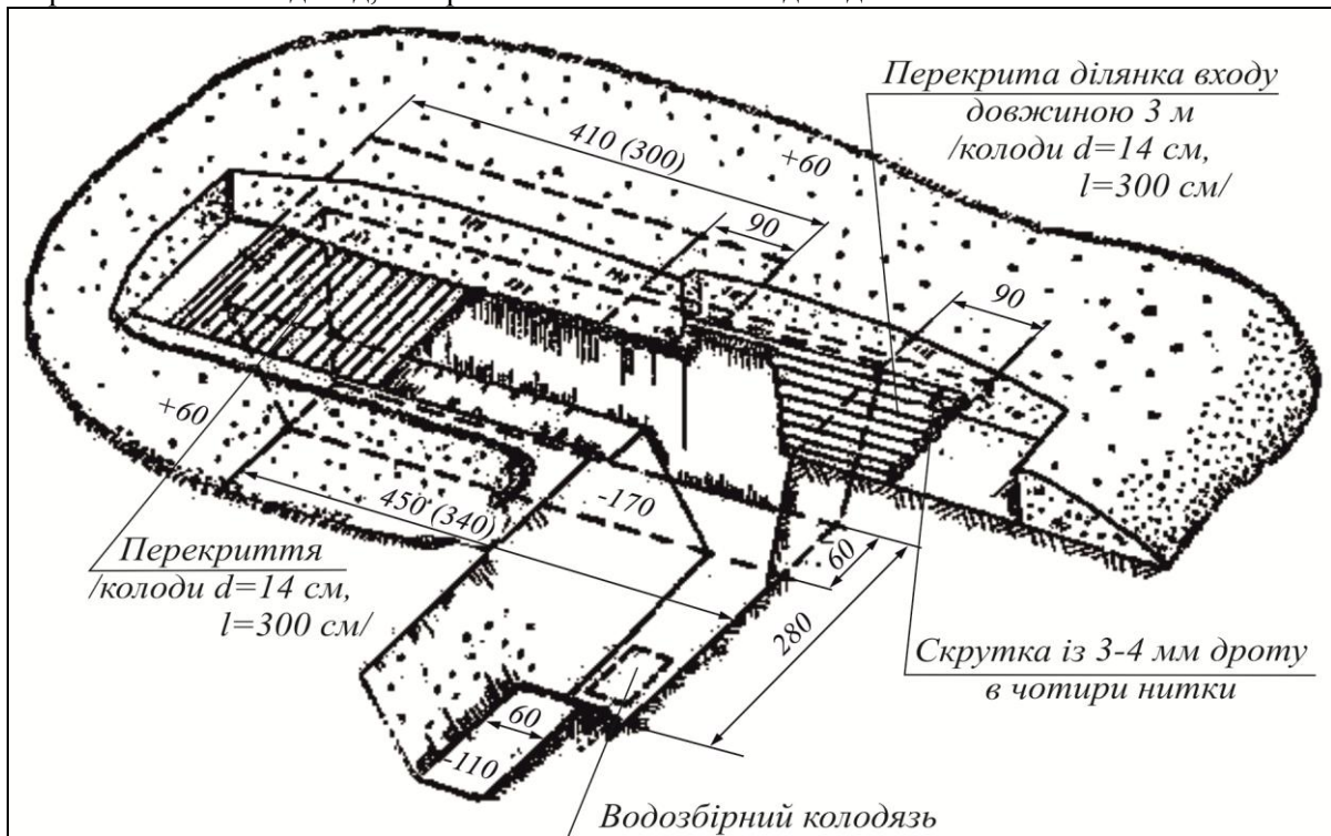
Рис. 14. Перекрита щілина на відділення (обслугову, екіпаж)
