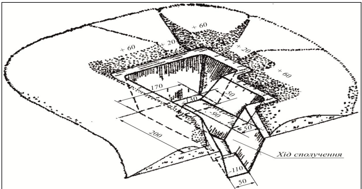
Рис. 16. Відкрите спорудження для спостереження командира взводу
