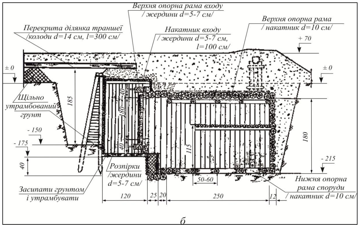
Рис. 15. Бліндаж безврубочної конструкції:
