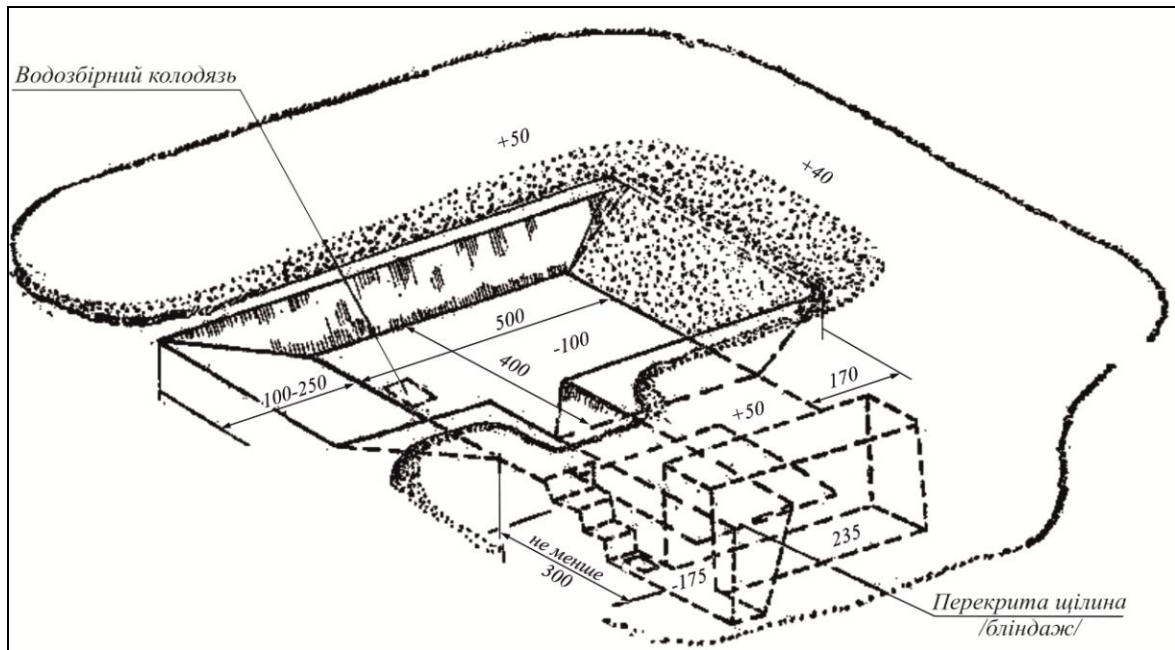
Рис. 12. Окоп для танка з круговим обстрілом
