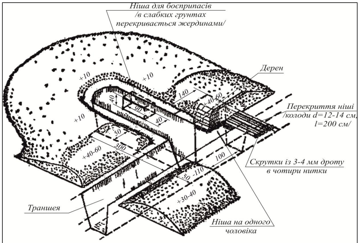
Рис. 8. Окоп для ручного протитанкового гранатомета
