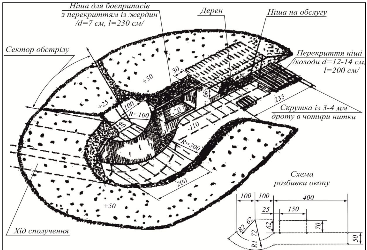
Рис. 10. Окоп для виробу 9К111 (9К115)
